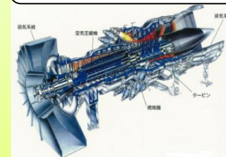
コンバインドサイクル発電用ガスタービン
