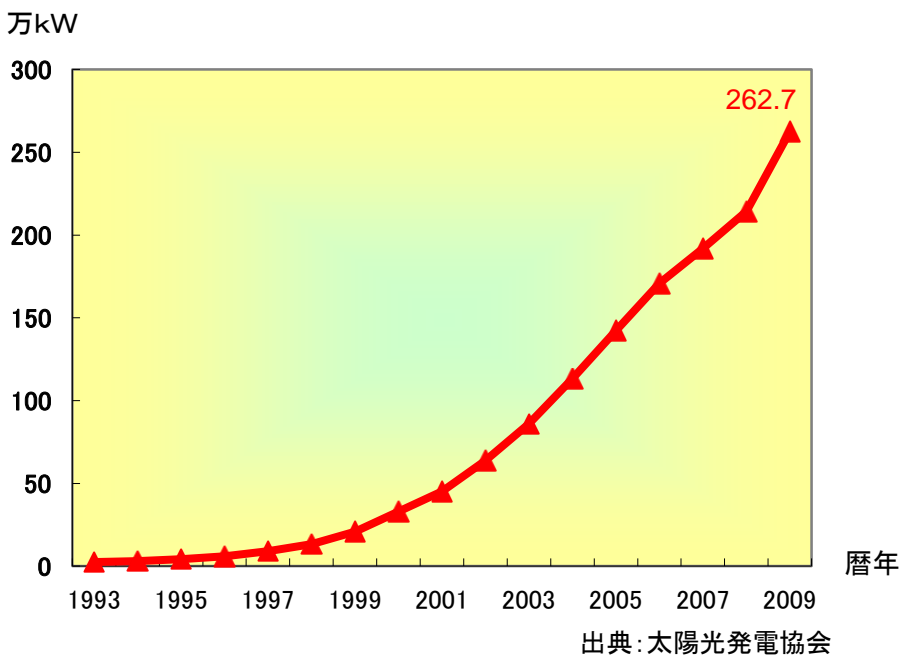
国内の太陽光発電累積導入量の推移
